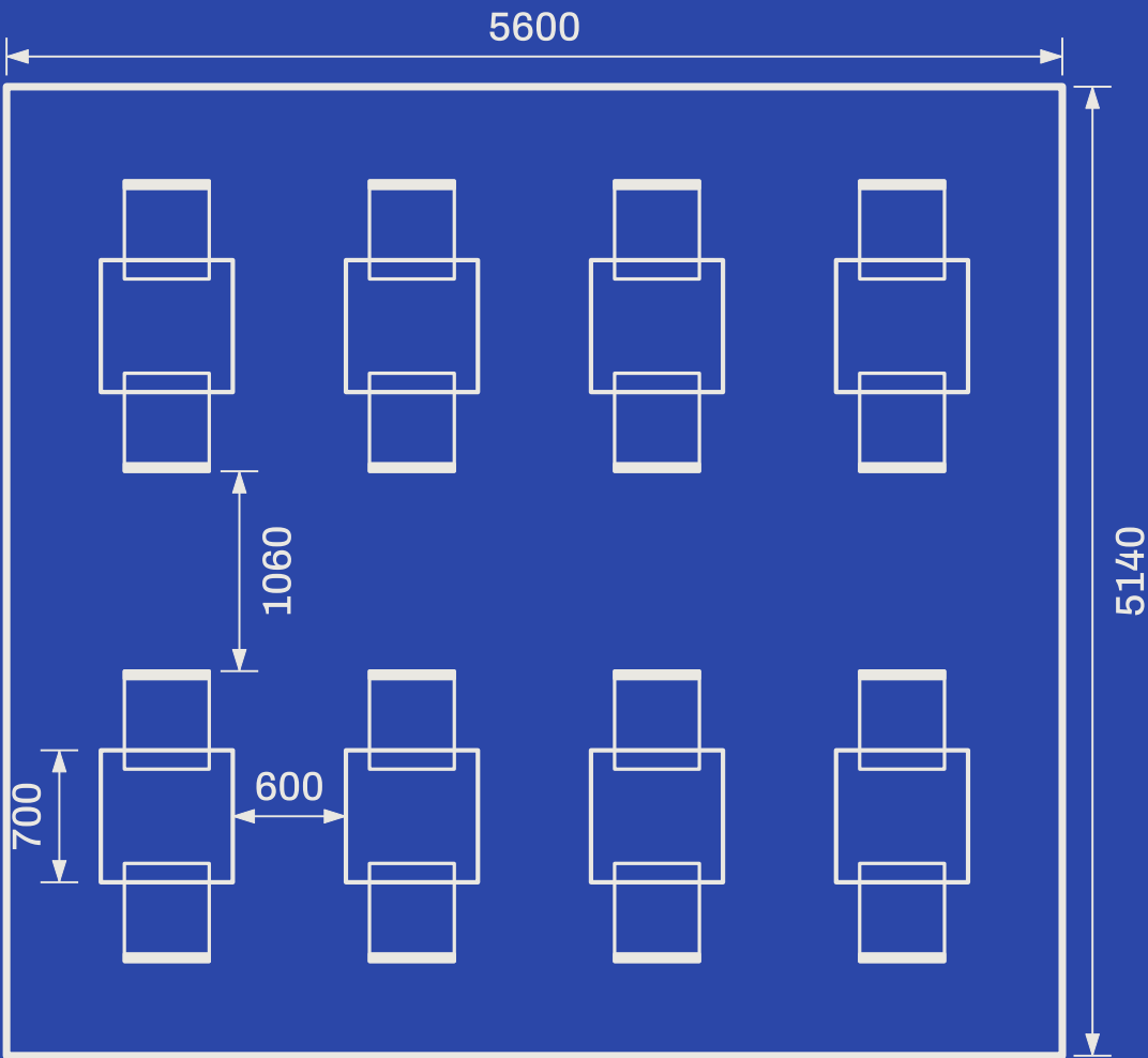
Esquisse d'implantation vue de dessus : 16 couverts sur 28,8 m², soit 1,8 m² par couvert ; 1 900 mm entre tables, 1 060 mm entre dossiers chaises rangées. Cotes en millimètres.
